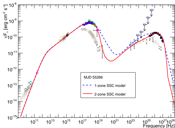
(b) MJD 55266.
