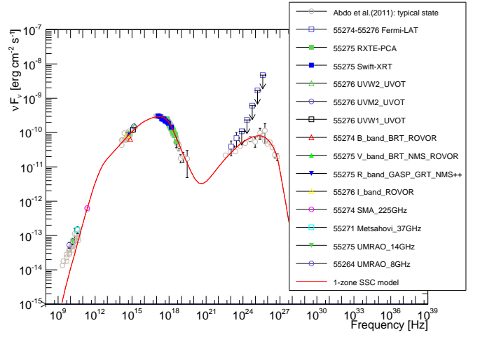
(d) MJD 55275.
