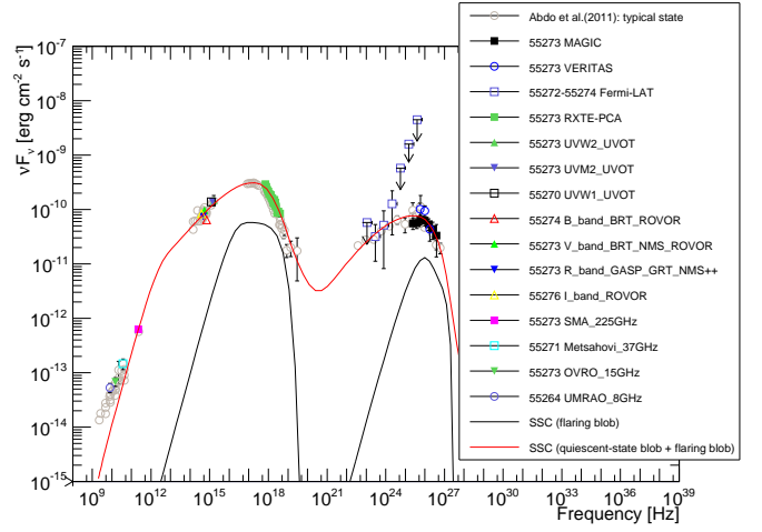
(b) MJD 55273.
