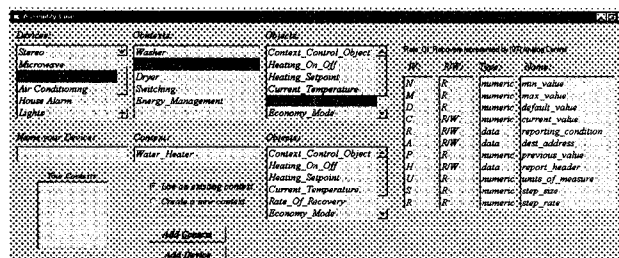
Fig: 2 CEBus Network Browser UI
